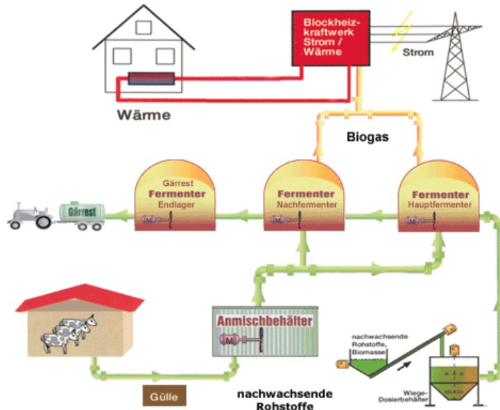
NawaRo-Anlage (Quelle: NEP GmbH & Co KG)
